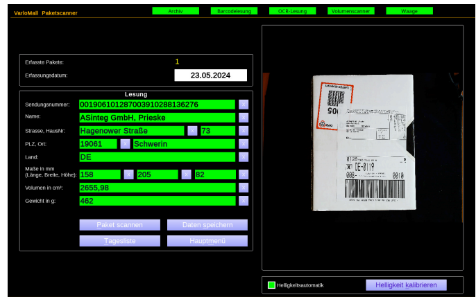
GUI-Beispiel
